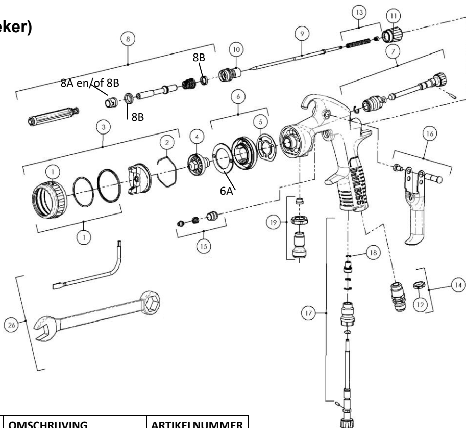
Art.nr. PRO-473 / 905284 pakkingset tbv luchtklepkooi PRO- 471/905282
